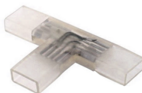
Ejemplos de empalmes para tiras de 220V RGB
